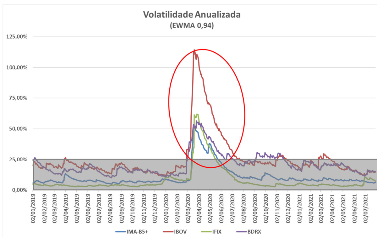
Gráfico 1 - Volatilidade Anualizada
