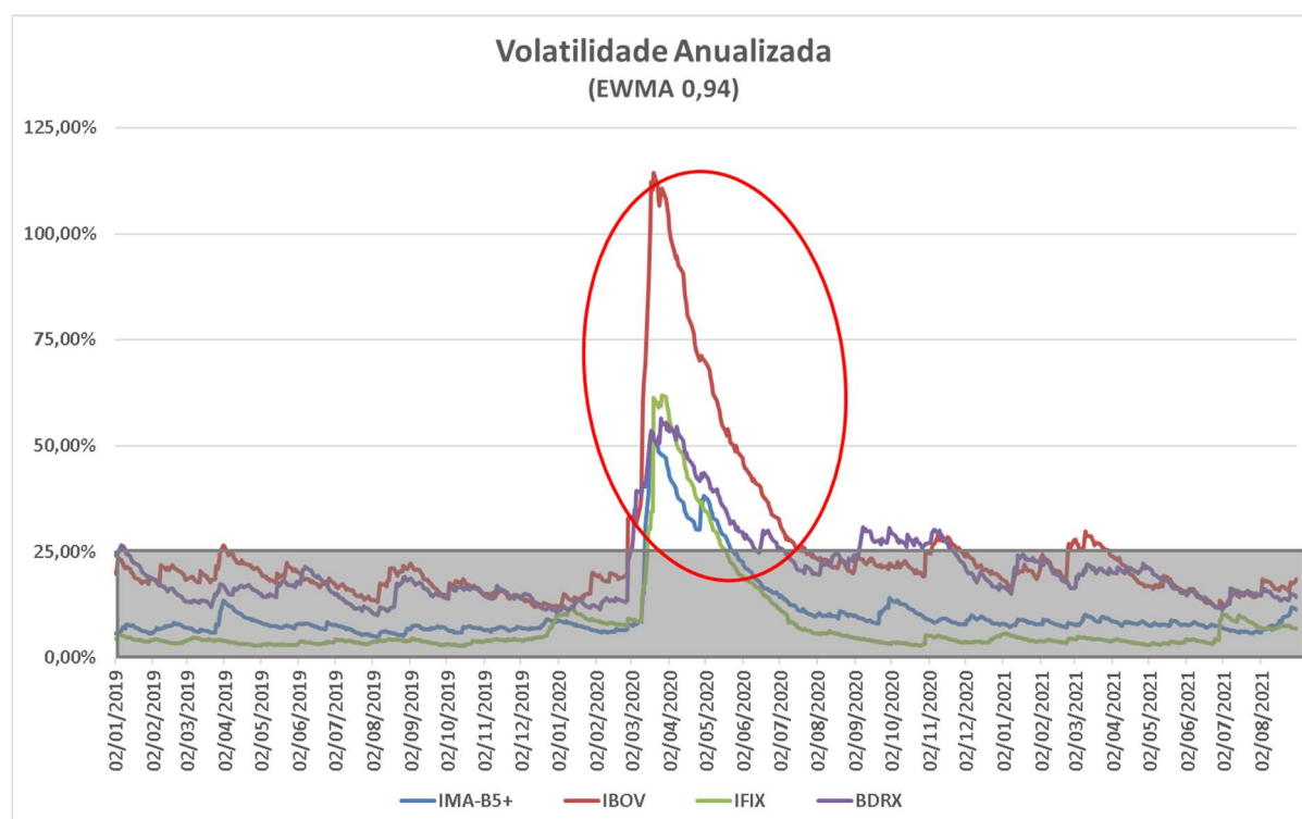
Gráfico 1 - Volatilidade Anualizada
