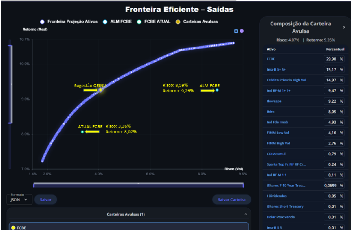
FIGURA 4 - Fronteira Eficiente e Carteiras Ótimas - Retornos Projetados para 5 anos e Volatilidade com janela de observação de 5 anos – FCBE
